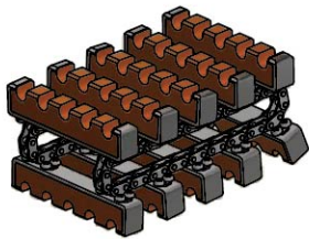
链式驱动组件
