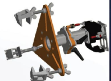
进枪导向装置
