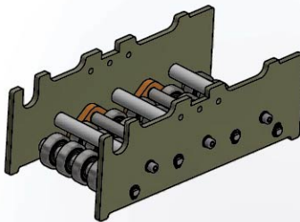
主机从动模块
